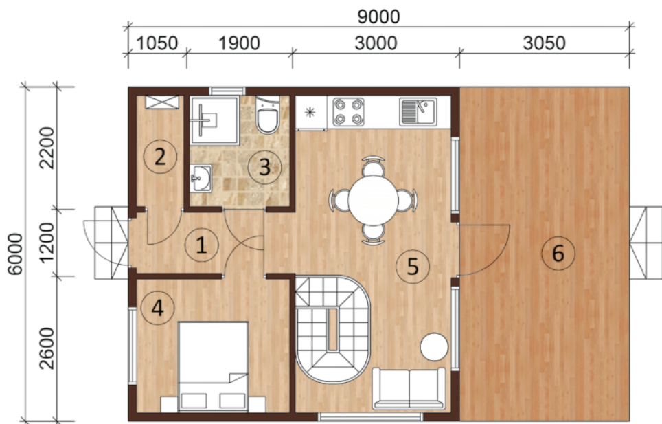
План 1 этажа
