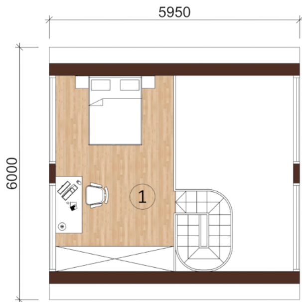
План 2 этажа
